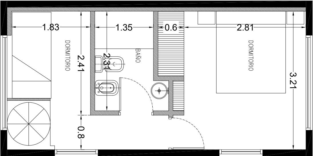
PLANTA ALTA
