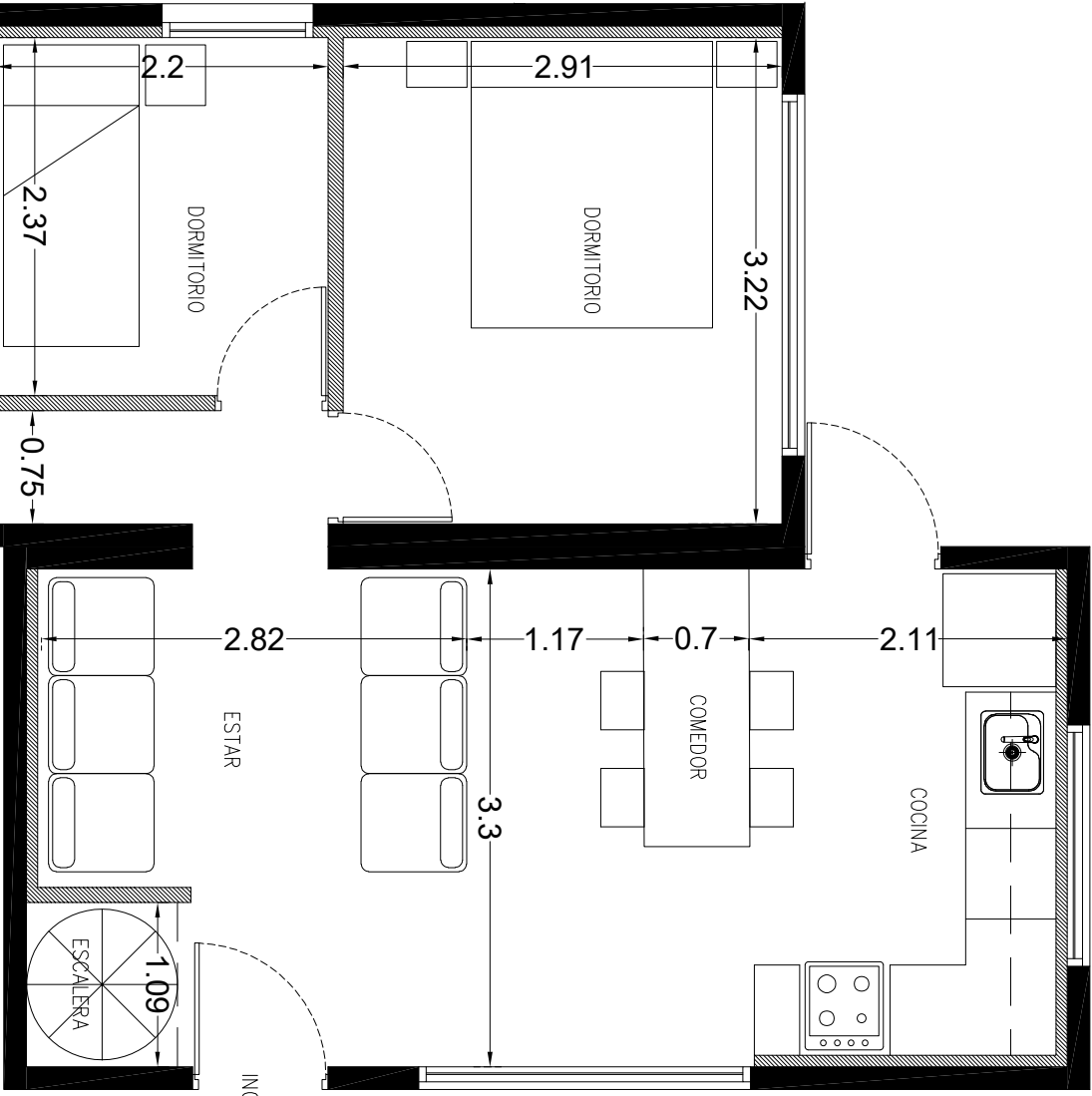
PLANTA BAJA
